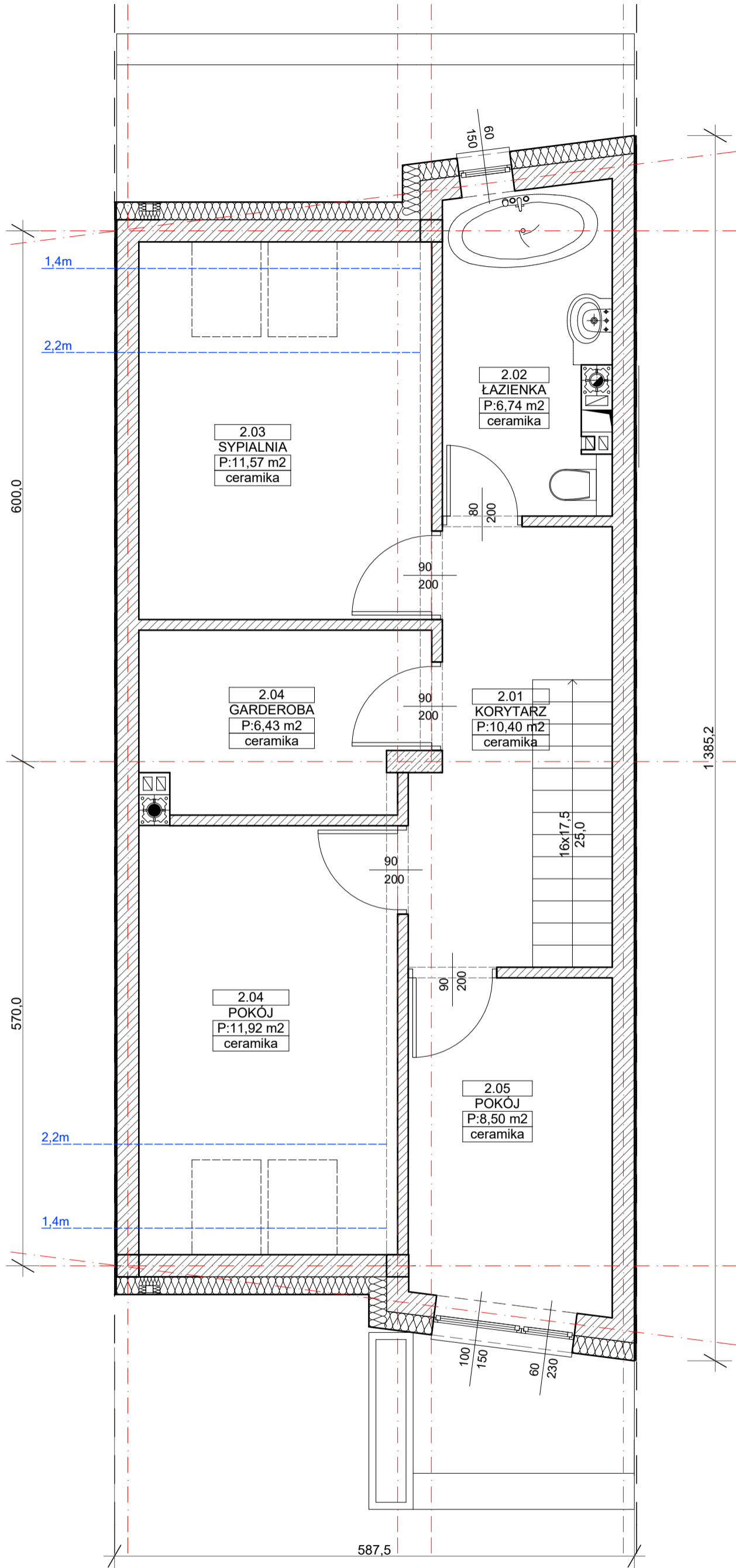
RZUT PODDASZA SEGMENT WYDŁUŻONY ŚRODKOWY
